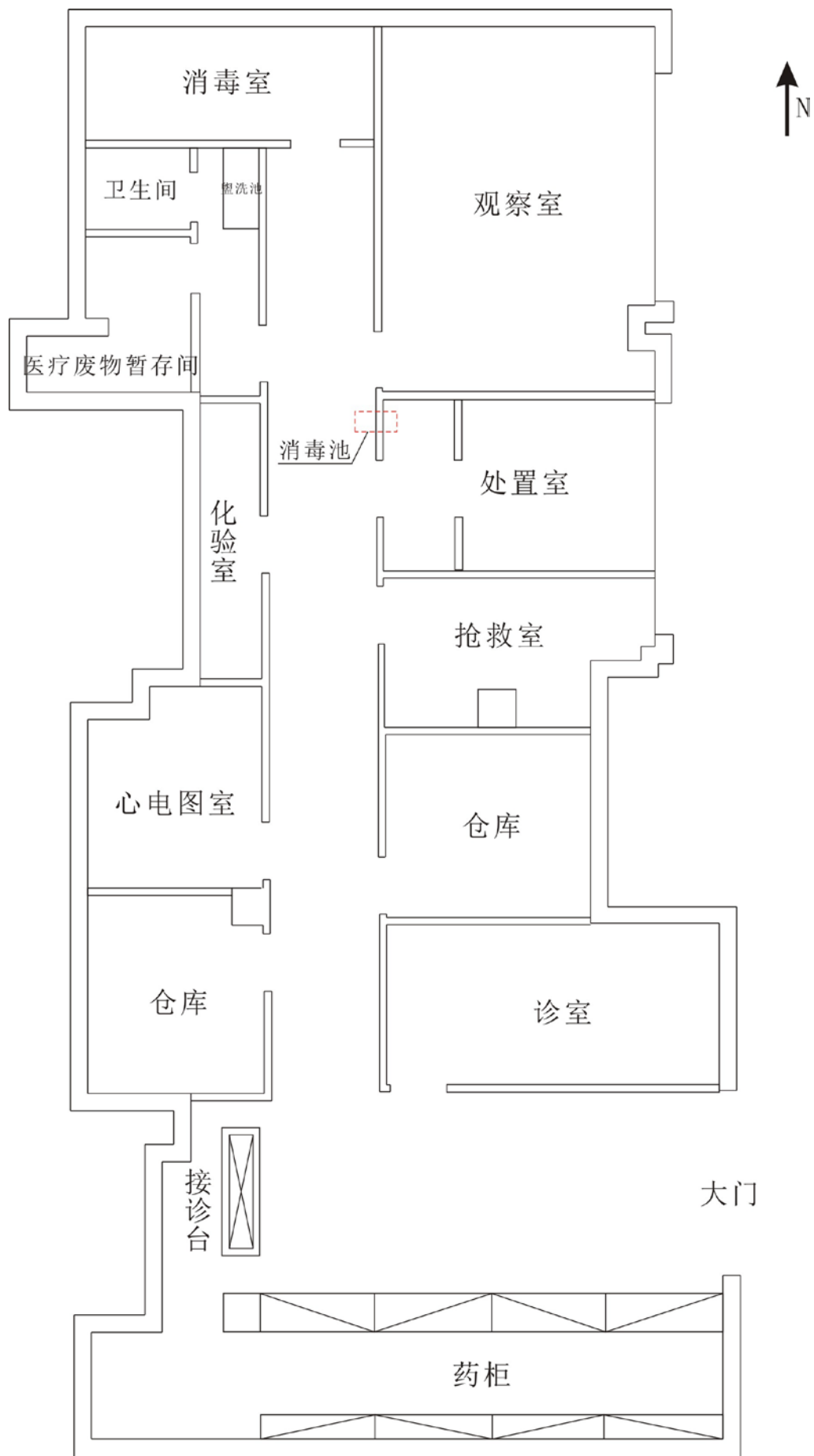
附图 2 建设项目平面布局图
